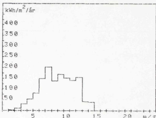
Mynd 11 b. Býtið av vindorkuni á eystri. Míðal fyri tíðarskeiðið 1974-78.
