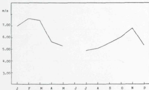
Mynd 4c. Mánaðarlig miðalvindferð í 1976.
