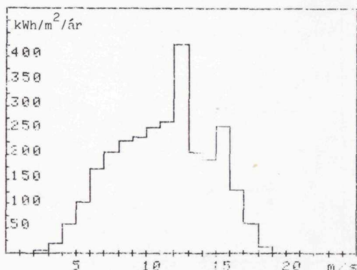
Mynd 11 d. Býtið av vindorkuni á suðri. Míðal fyri tíðarskeiðið 1974-78.
