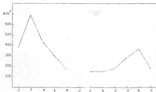
Mynd 6c. Mánaðarlig miðaleffekt í 1976.
