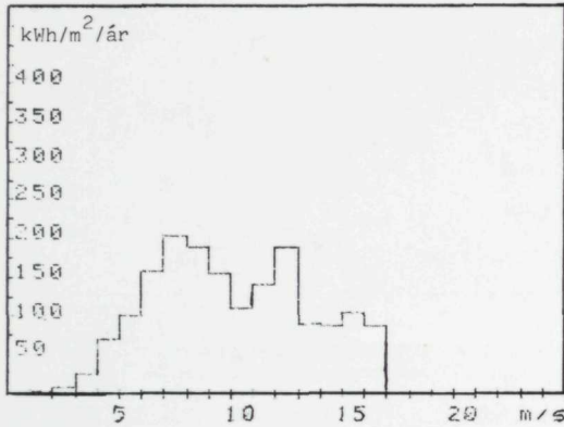
Mynd 11 g. Býtið av vindorkuni á útnyrðingi. Miðal fyri tíðarskeiðið 1974-78.
