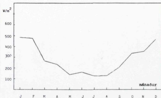
Mynd 7 Miðaleffektin pr. m 2 í vindinum einstöku mánaðirnar. Miðal fyrri tíðarskeiðið 1974-78.
