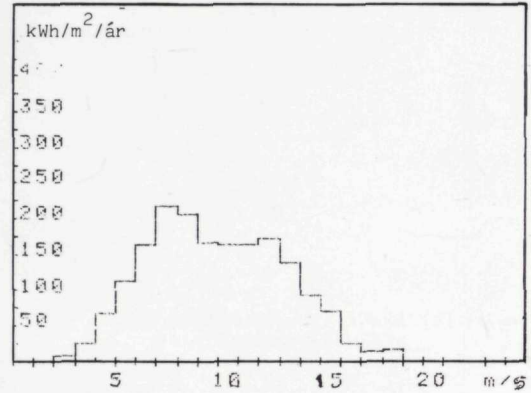
Mynd 11 h. Býtið av vindorkuni á norði. Miðal fyri tíðarskeiðið 1974-78.
