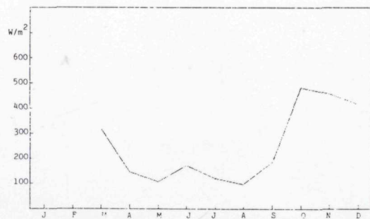
Mynd 6e. Mánaðarlig miðaleffekt í 1978.
