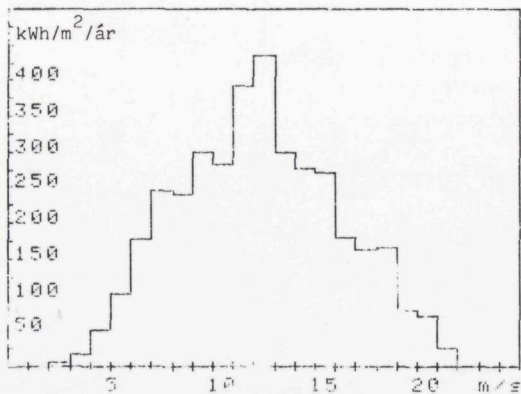
Mynd 11 e. Býtið av vindorkuni á útsynningi. Míðal fyri tíðarskeiðið 1974-78.
