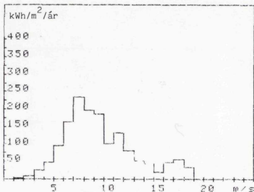
Mynd 11 a. Býtið av vindorkuni á landnyrðingi. Míðal fyri tíðarskeiðið 1974-78.
