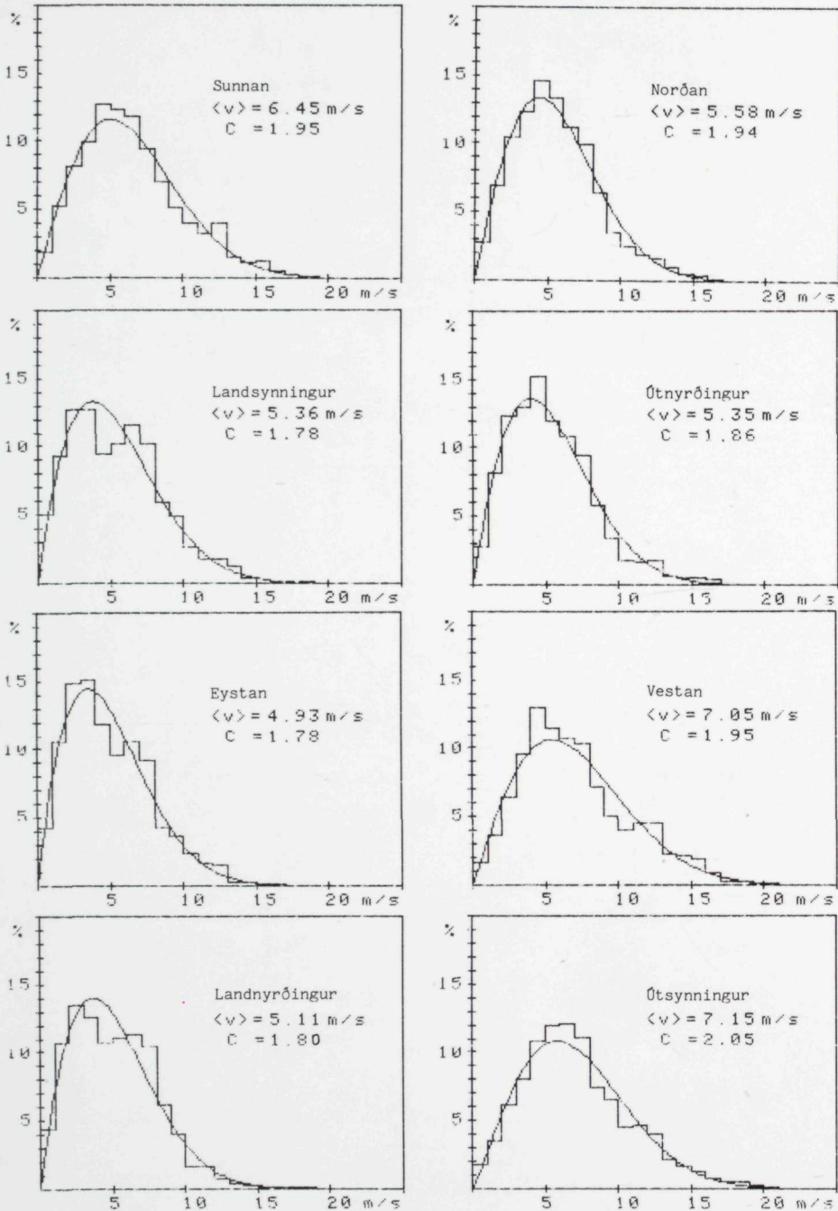
Mynd 8. Vindbýtió innan einstöku áttirnar. Miðal fyri tíðarskeiðið 1974-78. \langle v \rangle er miðalvindferðin og C er skap-parameturin í Weibull-býtinum.
