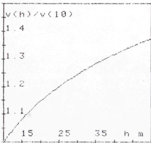
Mynd 1. Vindferðin í hæddini h í mun til vindferðina í 10 m hædd.
