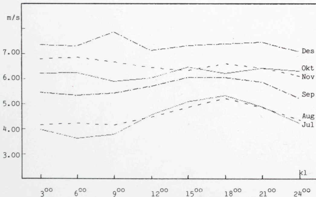
Mynd 2. Daglig broyting í miðalvindferðini. Miðal fyrí tíðar-skeiðið 1974-78.
