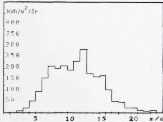
Mynd 11 i. Býtið av vindorkuni sum heild í tíðarskeiðinum 1974-78. Árliga miðalorkan var 2447 kWh/m²/ár.
