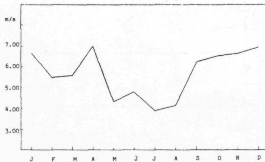
Mynd 4d. Mánaðarlig miðalvindferð í 1977.
