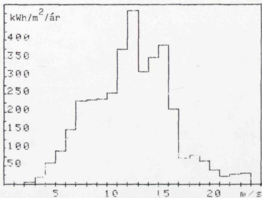
Mynd 11 f. Býtið av vindorkuni á vestri. Míðal fyri tíðarskeiðið 1974-78.
