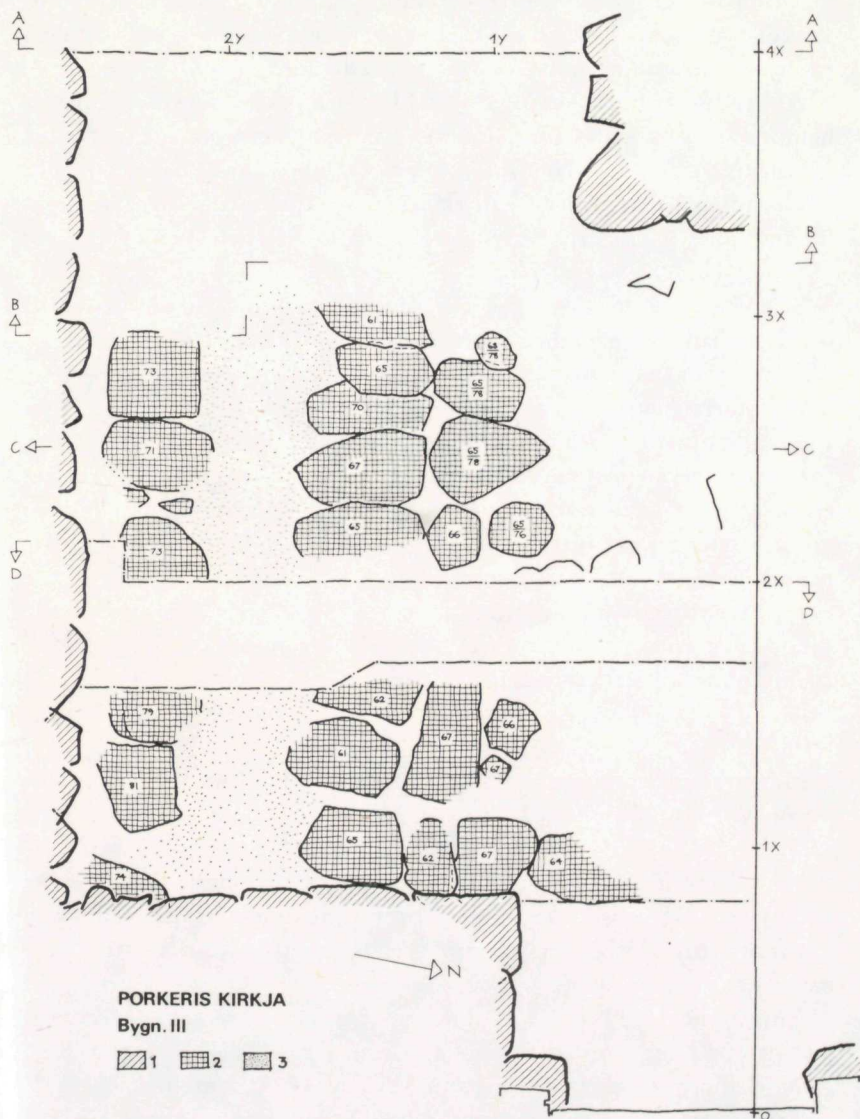
Mynd 4. Flatatekning 2, Bygn. III. Teknlýsing : 1. Grund og miðlaðing á núverandi kirkju. 2. Leivdir av veggj og grund á bygn. III. 3. Fylla í veggj á bygn. III.
