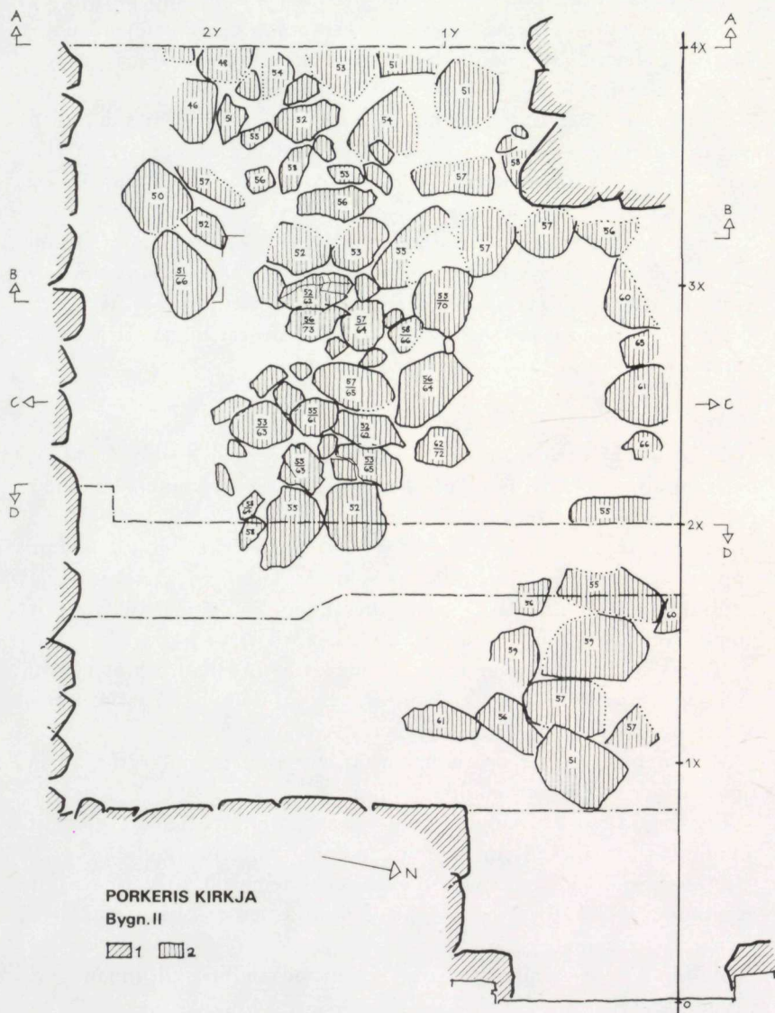
Mynd 3. Flatatekning 1, Bygn. II. Teknlýsing: 1. Grund og miðlaðing á núverandi kirkju. 2. Leiðir av gólvi í bygn. II.
