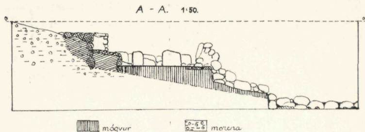
MYND 5. Tvörskurður A—A á flatatekningini (mynd 4) við öllum veggjunum aftanfyri skurðin innteknaðum. Cross-section A—A on the plane.
