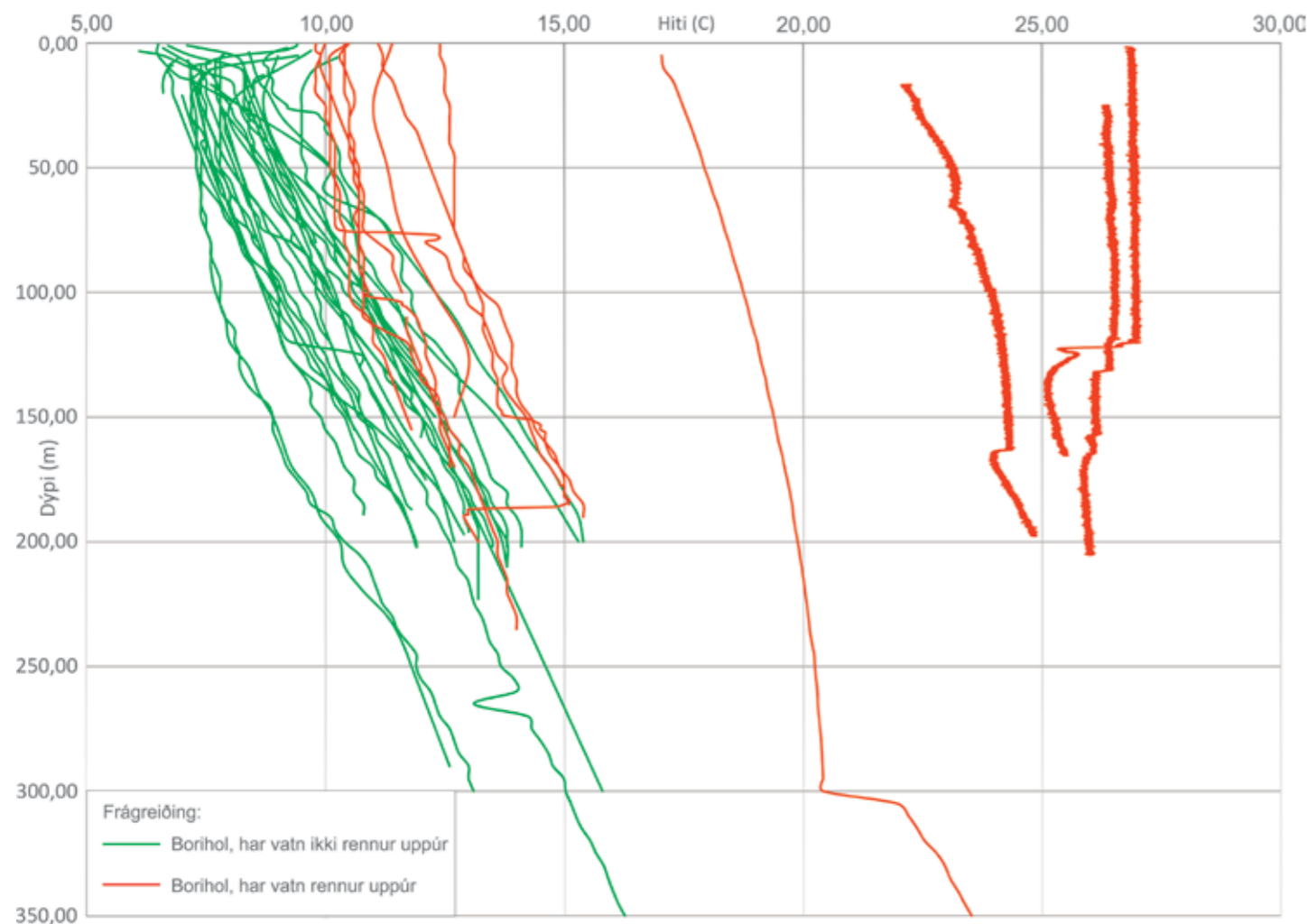
Mynd 5. Málða hitastigið pr. dýpi í vatninum á ymiskum boringum í Føroyum. Reyðu kurvarnar vísa mátingar av boriholum, har vatn rennur út av sær sjálvum (artesisisk hol), meðan grønu kurvarnar vísa borihol, har vatn ikki rennur út.
