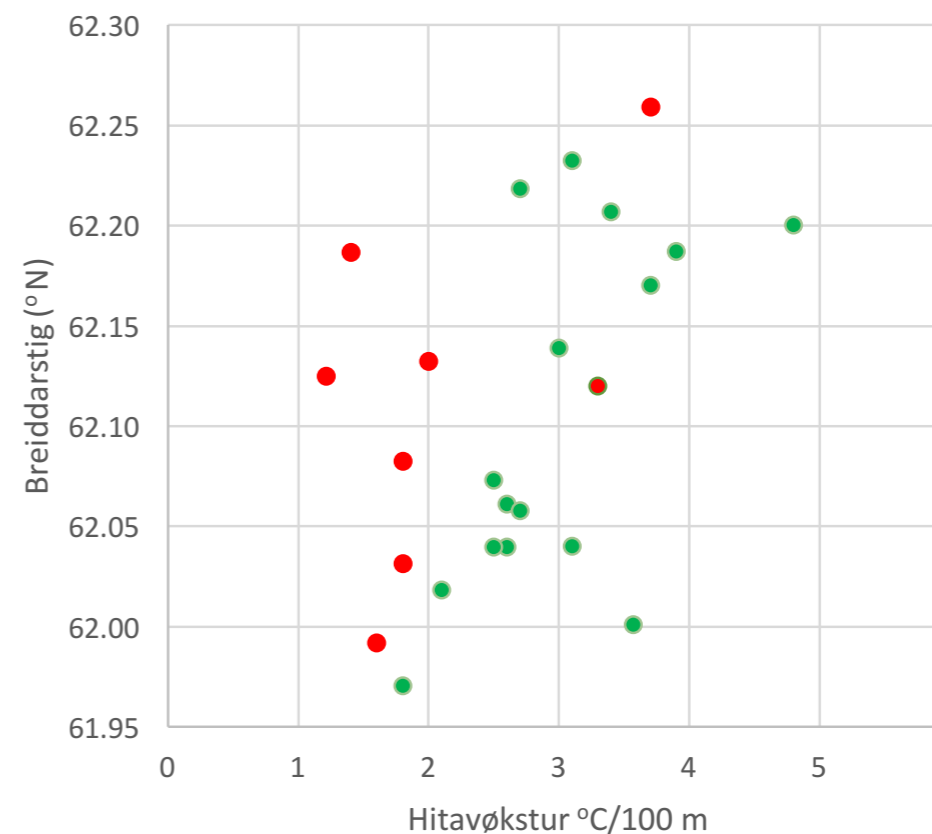
Mynd 6. Jarðhitavøkstur (x-ásin) í ymiskum boriholum í norðara parti av Føroyum (y-ásin). Teir reyðu prikkarnir vísa hitavøksturin í boriholum, har vatn rennur út, meðan teir grønu prikkarnir vísa hitavøksturin í boriholum, har einki vatn rennur út. Breiddarstigið 62,1°N á y-ásinum er á leið, har Kaldbaksbotnur er.
