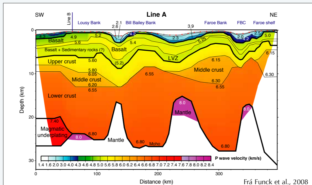
Mynd 5: Landgruns-verkætlanin fekk til vegar hópin av nýggjum havbotnsdátum. Myndin vísir ein skurð gjøgnum jarðarskorpuna sunnan fyri Føroyar frá seismiskum dátum.
